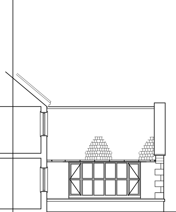
Elevation E
